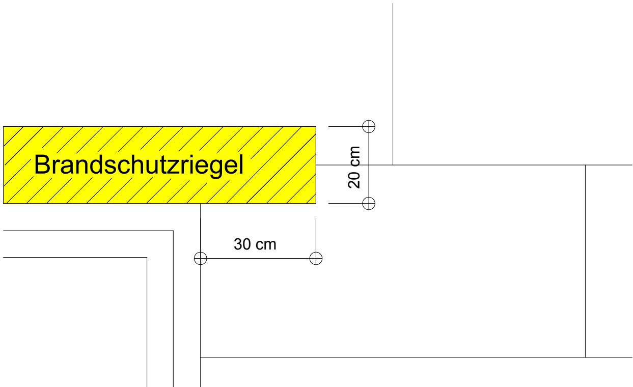
a) Brandschutzriegel Anordnung in Höhe des Fenstersturzes
