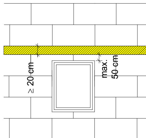
b) Brandschutzbänderole Anordnung über der nächsten Dämmplattenschar
