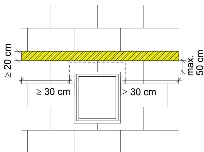
d) Anordnung des Brandschutzschottes bei einer Sonnenschutzeinrichtung
