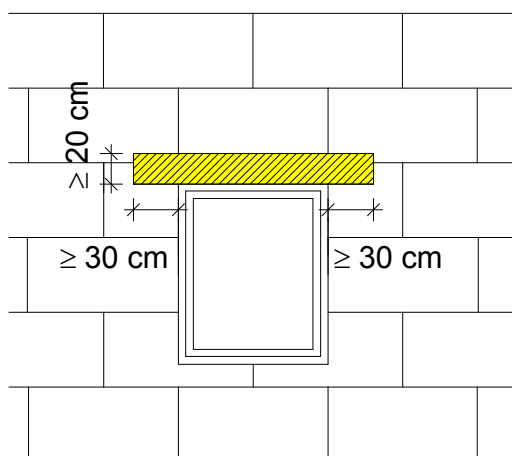
a) Brandschutzriegel Anordnung in Höhe des Fenstersturzes
