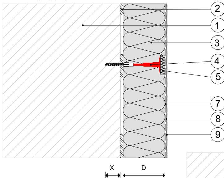
a) Baunit SchraubDübel Speed mit Rondelle
