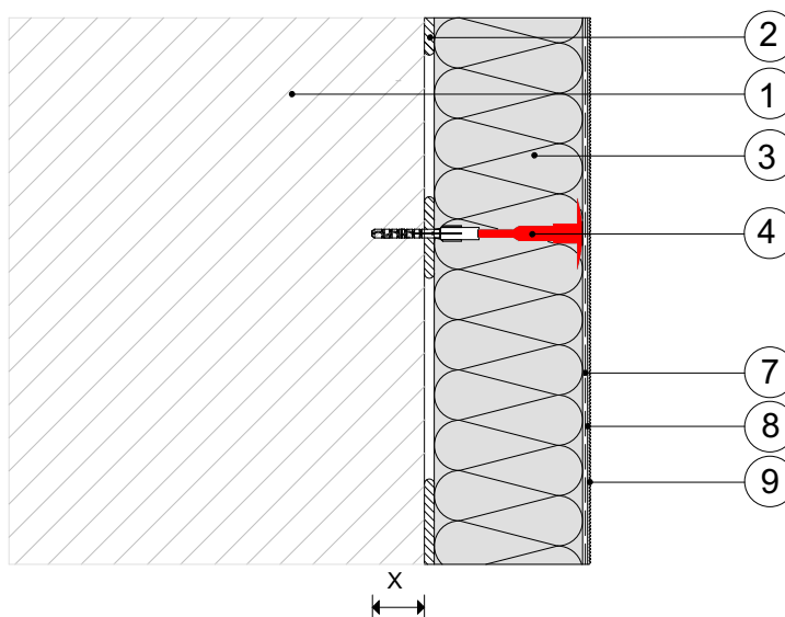
b) Baunit SchraubDübel Speed oberflächenbündig
