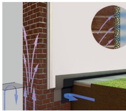
Saniertes Mauerwerk
