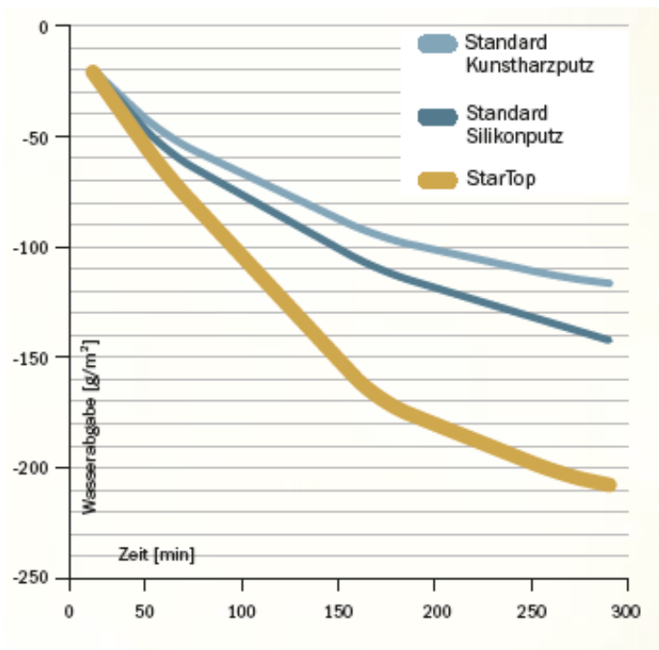
Foto_Baumit_StarTop_02.jpg: StarTop im Vergleich: 100% höhere Wasserabgabe als ein Standard-Kunstharzputz und 66% höhere Wasserabgabe als ein Standard-Silikonputz.
